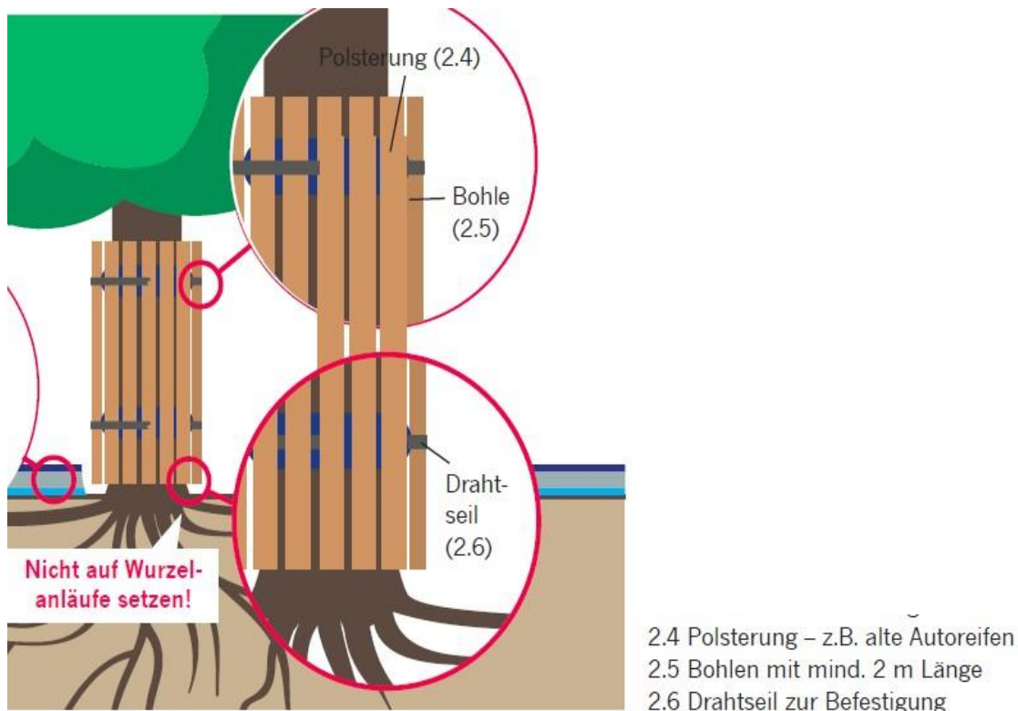
Abbildung 13: Skizze für einen Stammschutz, um Stammschäden zu verhindern (Quelle: Merkblatt des Gartensamtes der Stadt Düsseldorf)
