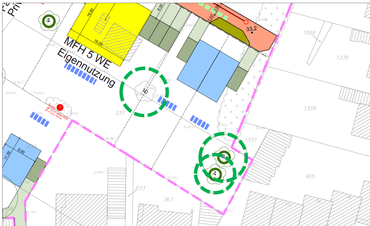
Abbildung 5b: Lage der Betrachtungsgruppe 3 – Bäume V-Z, ZA und Betrachtungsgruppe 4 – Bäume 6-7, 10 innerhalb der Planung / Auszug Erschließungsplanung (Büro bPlan, Essen / Stand 22. Juni 2023)
