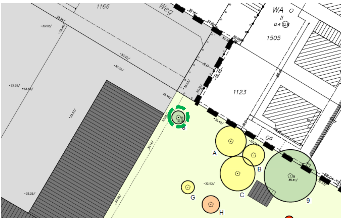
Abbildung 7a: Lage des Einzelbaums 8 im Plangebiet / Auszug Lageplan „Baumkataster / -bewertung“ (Normann / Stand 19. Oktober 2021)
