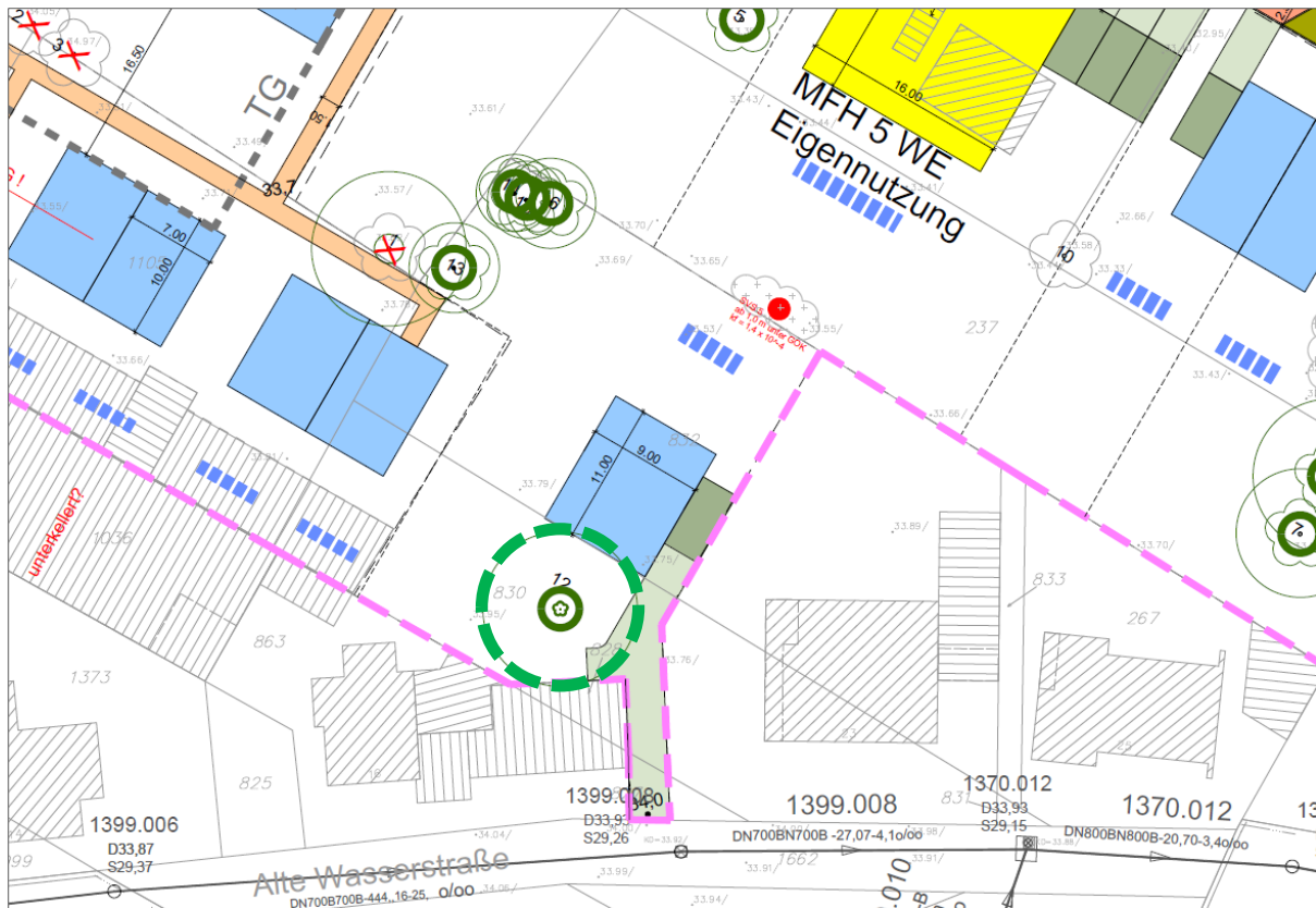
Abbildung 9b: Lage des Einzelbaums 12 innerhalb der Planung / Auszug Erschließungsplanung (Büro bPlan, Essen / Stand 22. Juni 2023)
