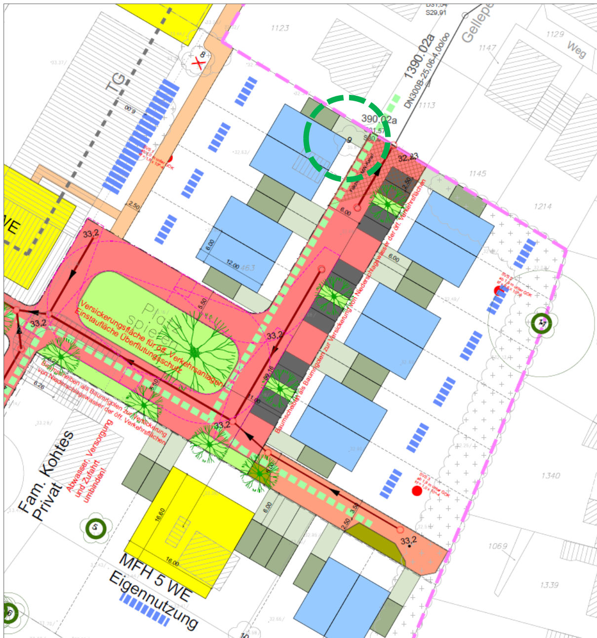
Abbildung 4b: Lage der Betrachtungsgruppe 2 – Bäume 9, A-U, ZB innerhalb der Planung / Auszug Erschließungsplanung (Büro bPlan, Essen / Stand 22. Juni 2023)
