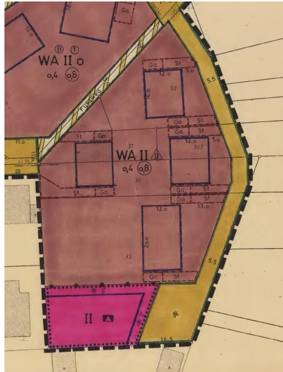
Ausschnitt aus der 1. Änderung zum Bebauungsplan Nr. 136
